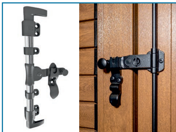
CHIUSURA SUPERIORE
